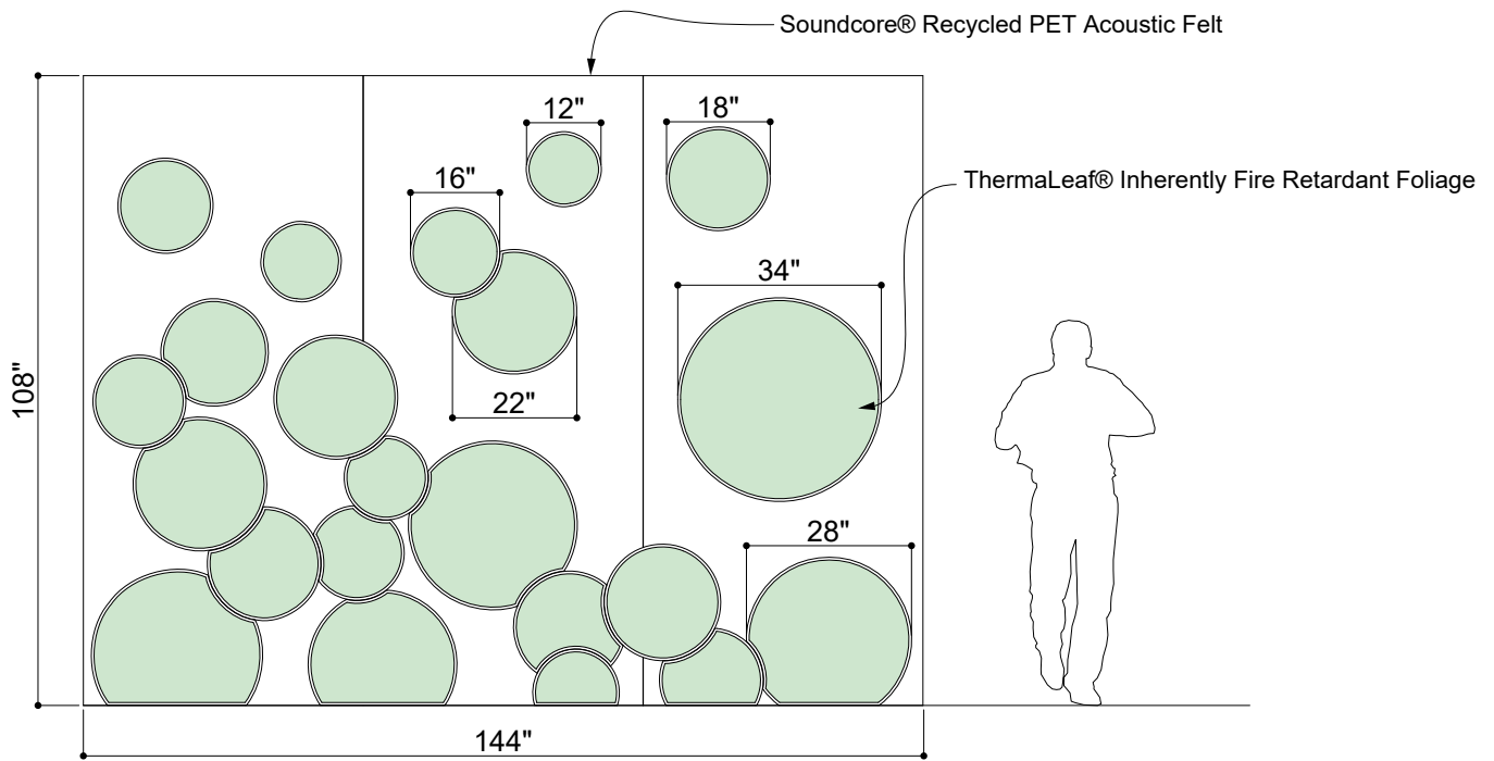
① ELEVATION 1
